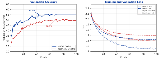
Fig. 2: 训练动态。左：验证准确率。右：损失曲线。
