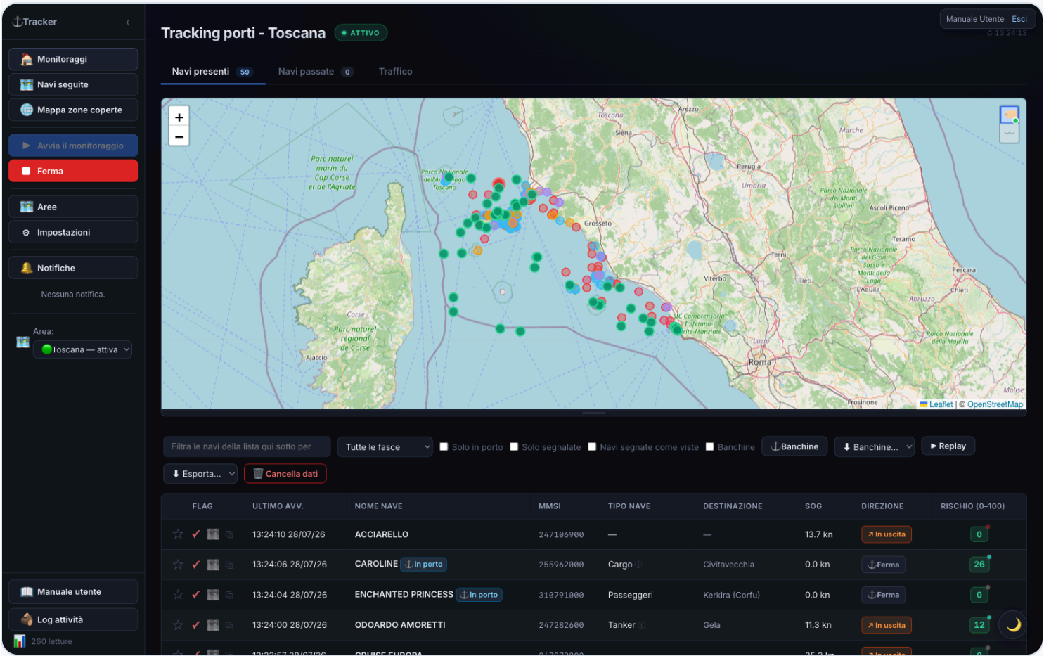
Scheda Navi presenti: mappa con i marker delle navi colorati per rischio e tabella dettagliata sotto.
