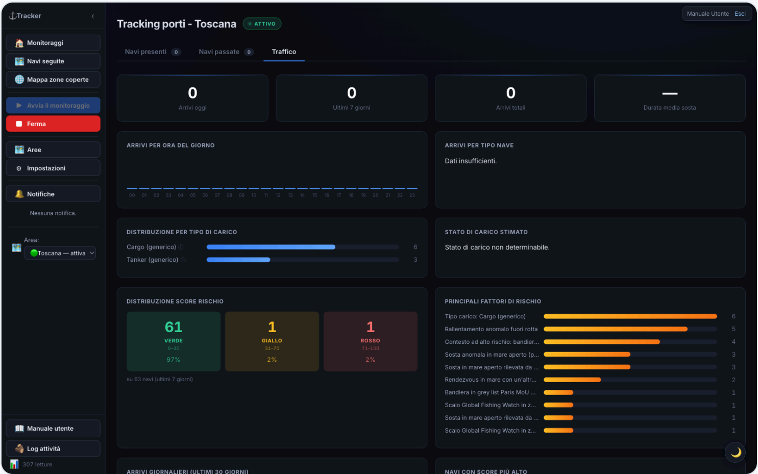
Scheda Traffico: schede statistiche in alto e grafici su arrivi per ora, tipo nave, distribuzione rischio e andamento giornaliero.
