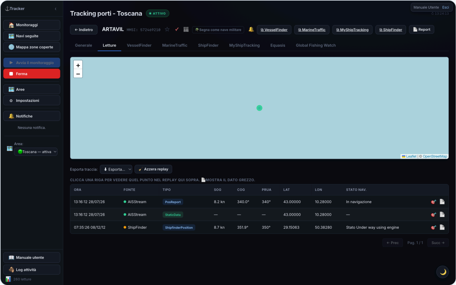
Dettaglio nave — tab Letture: mappa con traccia/replay fissa in alto e tabella paginata delle letture AIS.
