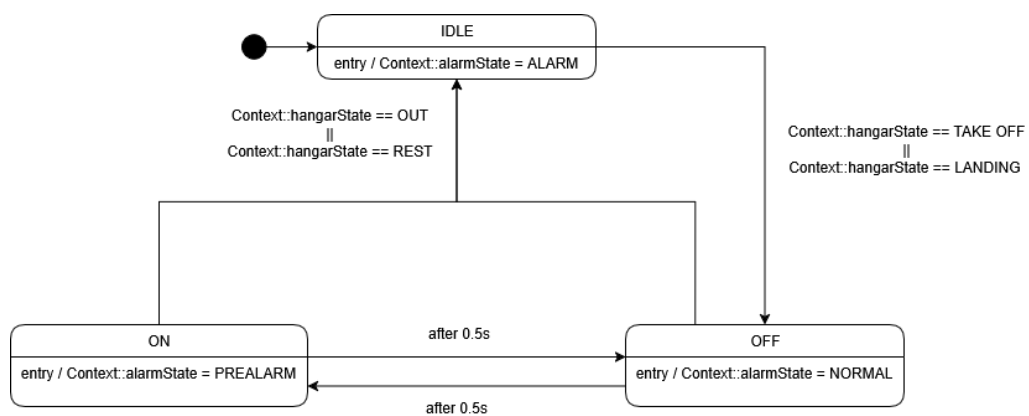
Figura 3.4: Macchina a stati del blinking del led
