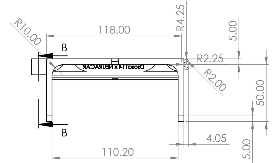
Vista Trasera
