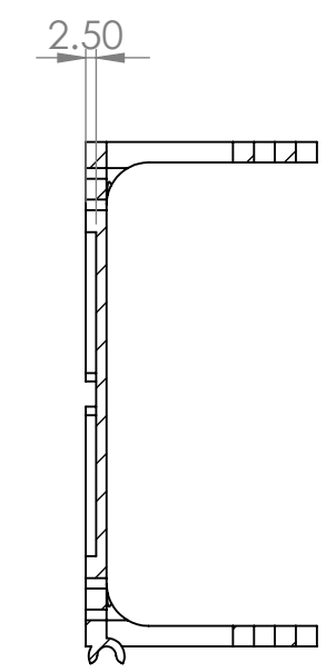
SECCIÓN C-C
