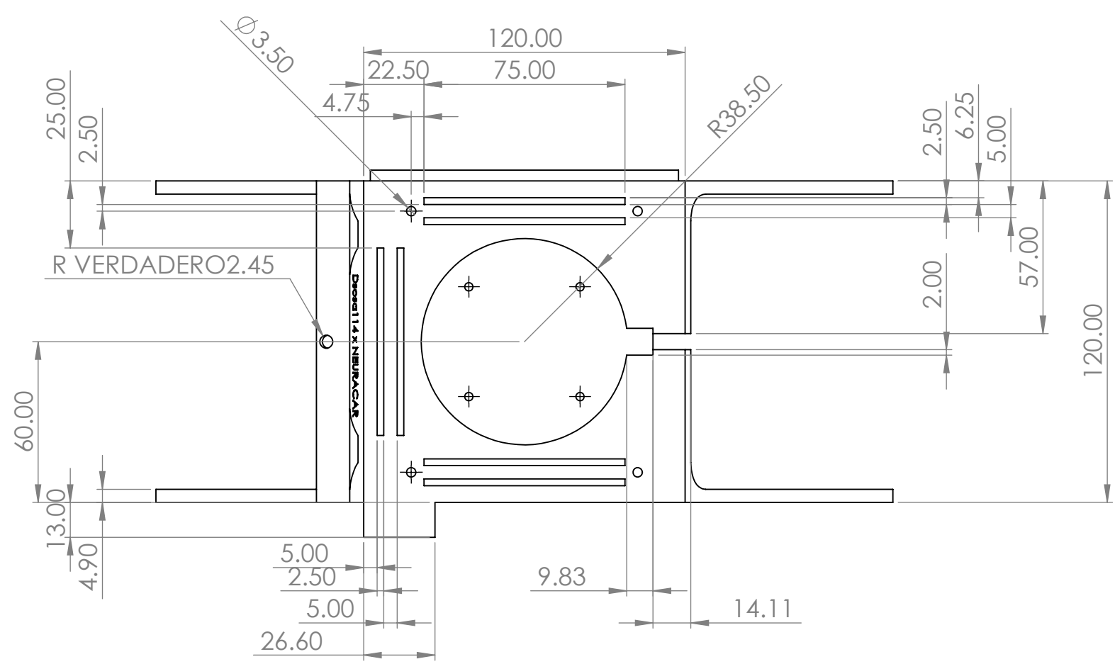
Vista Superior
