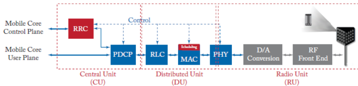
Εικόνα 3-5 Κατανεμημένο RAN σε CU, DU και RU
