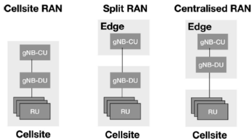
Εικόνα 3-9 Επιλογές ανάπτυξης NG-RAN
