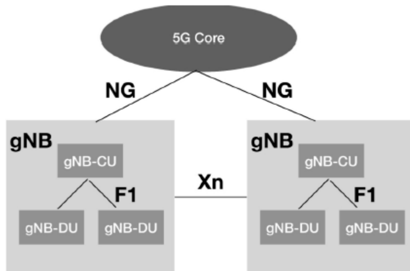
Εικόνα 3-8 NodeB επόμενης γενιάς (gNB)
