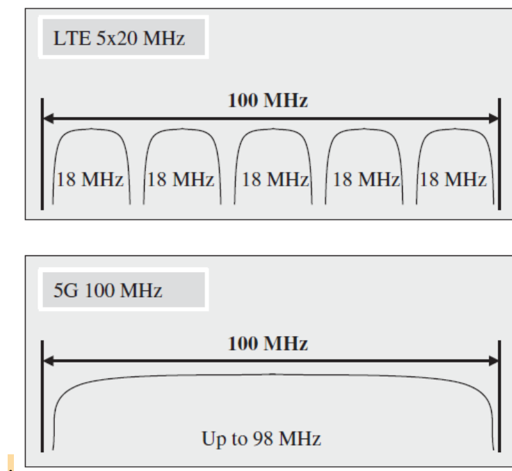
Εικόνα 2-3 Συνάθροιση φορέων 4G, φορέα 5G Πηγή [1]
