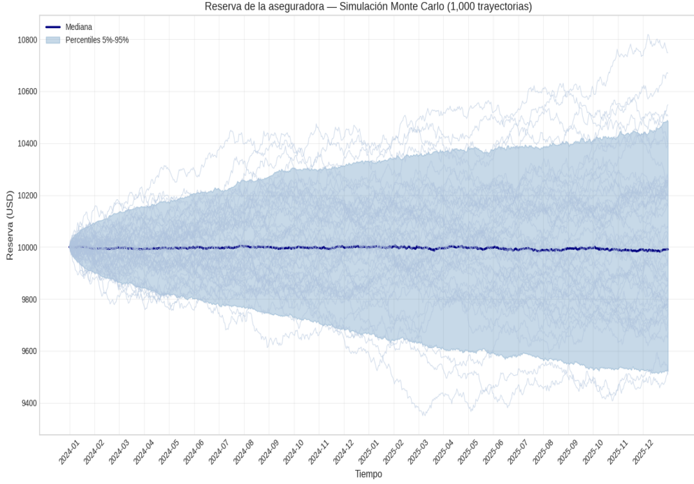
Figura 7.2: Metodo de Milstein con difusión y saltos aplicados al modelo de Cramér–Lundberg con difusión y saltos, adaptado específicamente para aseguradoras de viviendas.
