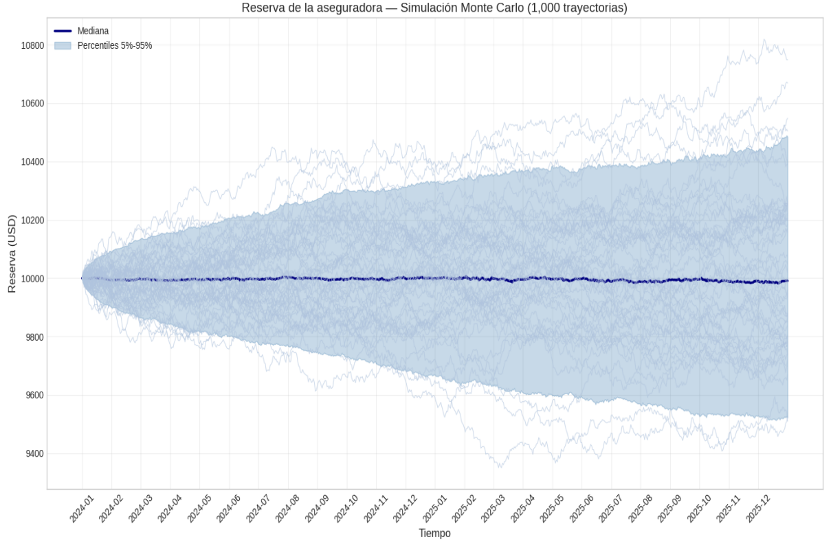
Figura 7.2: Metodo de Milstein con difusión y saltos aplicados al modelo modelo de Cramér–Lundberg con difusión y saltos, adaptado específicamente para aseguradoras de viviendas.
