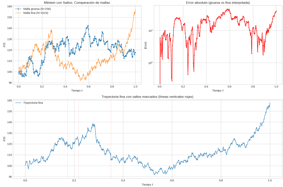
Figura 7.1: Metodo de Milstein con difusión y saltos aplicados al modelo modelo de Cramér–Lundberg con difusión y saltos, adaptado específicamente para aseguradoras de viviendas.
