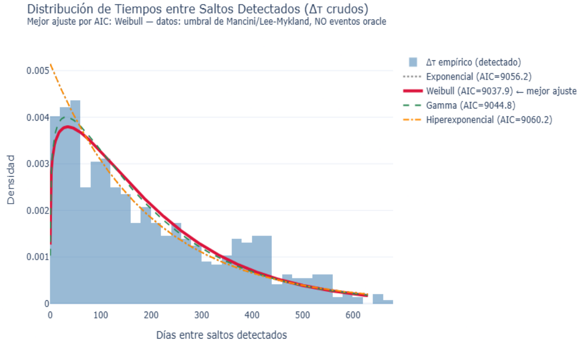
Figura 9.5: Histograma de \Delta\tau crudo (días) con las cuatro familias ajustadas superpuestas; Weibull resaltada como mejor ajuste por AIC.
