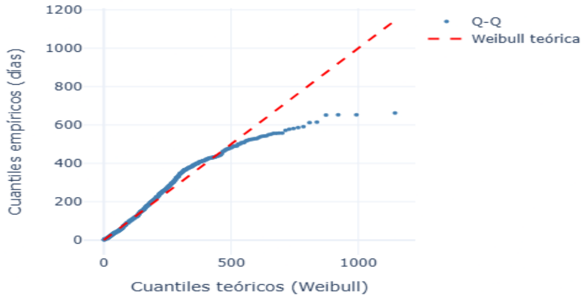
Figura 9.6: Q-Q plot de \Delta\tau empírico contra la Weibull ajustada ( k = 1.151 , \theta = 203.9 ).
