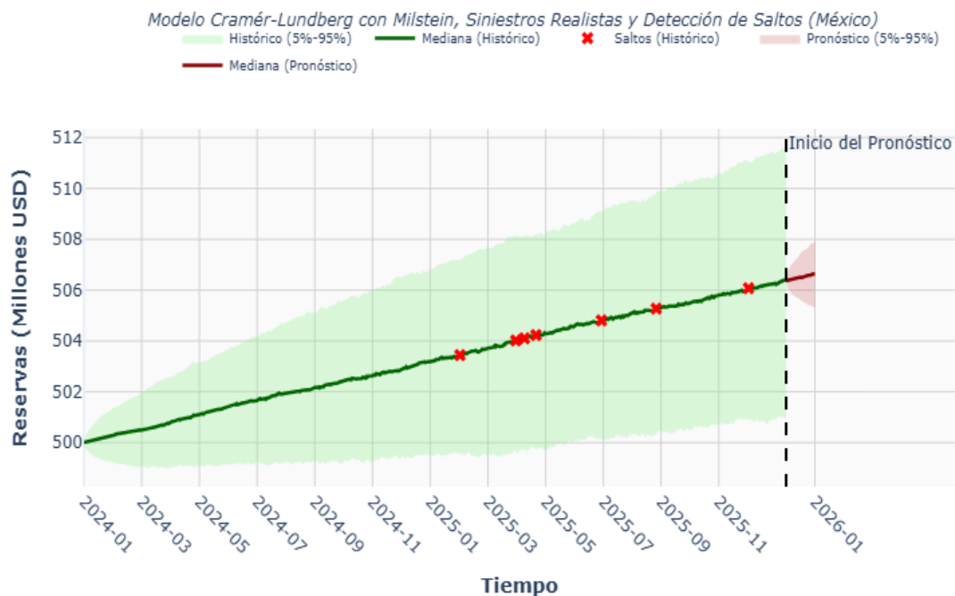
Figura 7.1: Trayectorias implementadas por el m3todo Milstein, medianas e intervalos de confianza 90 % (5 %-95 %) para ambos esquemas. Los marcadores ✕ (rojos) y ★ (azules) indican saltos detectados en las medianas hist3rica y de pron3stico, respectivamente. La l3nea vertical discontinua marca el inicio del pron3stico (enero 2026).
