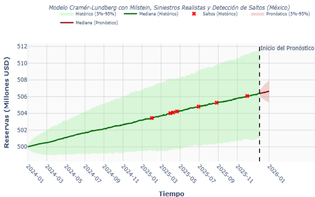
Figura 7.3: Trayectorias implementadas por el método Milstein, medianas e intervalos de confianza 90 % (5 %-95 %) para ambos esquemas. Los marcadores × (rojos) y ★ (azules) indican saltos detectados en las medianas histórica y de pronóstico, respectivamente. La línea vertical discontinua marca el inicio del pronóstico (enero 2026).
