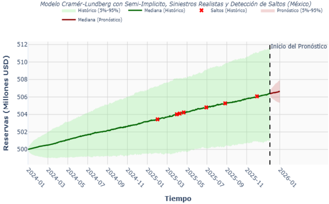
Figura 7.4: Trayectorias implementadas por el método Semi-Implicito, medianas e intervalos de confianza 90 % (5 %-95 %) para ambos esquemas. Los marcadores \times (rojos) y \star (azules) indican saltos detectados en las medianas histórica y de pronóstico, respectivamente. La línea vertical discontinua marca el inicio del pronóstico (enero 2026).
