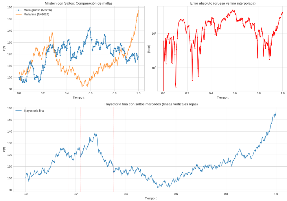
Figura 7.1: Metodo de Milstein con difusión y saltos aplicados al modelo modelo de Cramér–Lundberg con difusión y saltos, adaptado específicamente para aseguradoras de viviendas.
