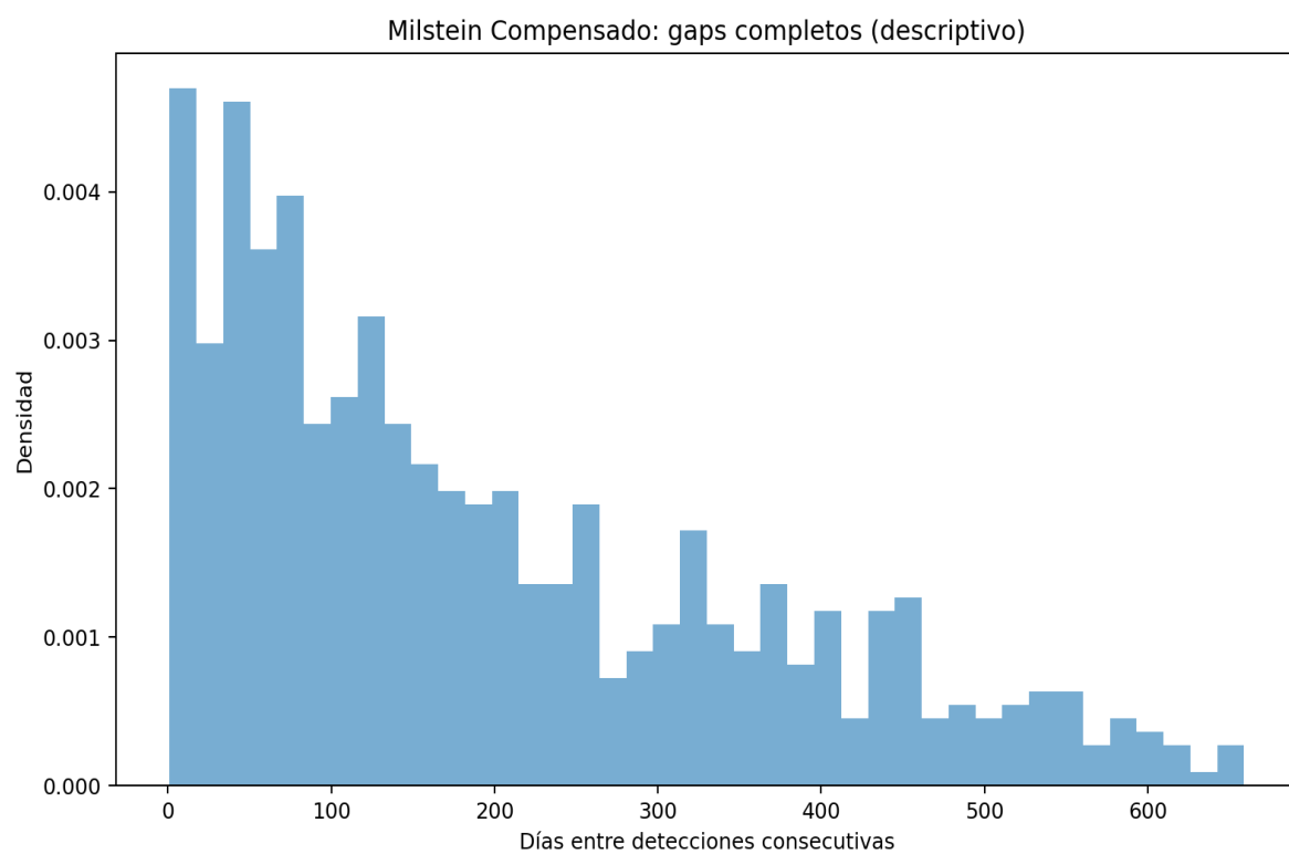
Figura 9.9: Histograma de gaps completos para Milstein compensado.
