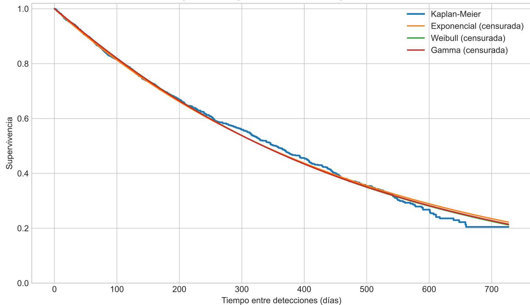
Milstein Compensado: supervivencia de los tiempos entre detecciones
