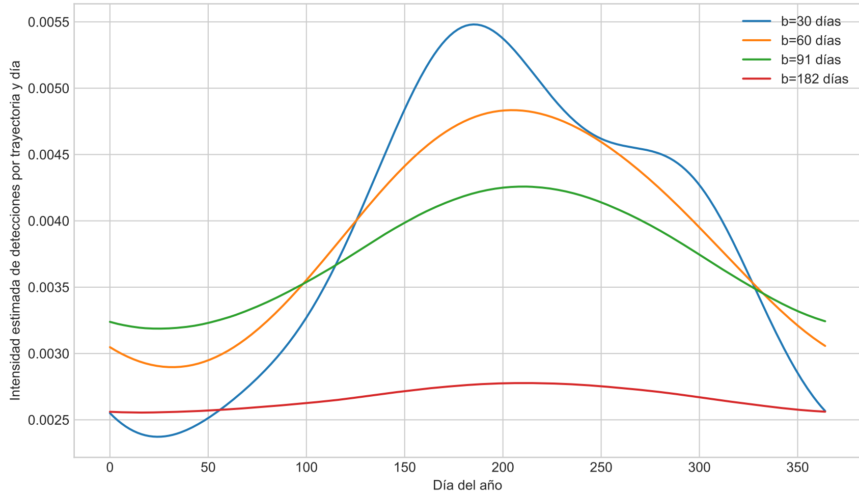
Milstein Compensado: sensibilidad del suavizado de intensidad
