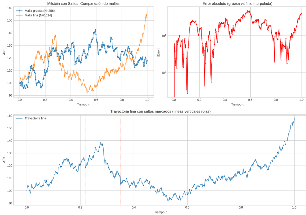
Figura 7.1: Comparación del método de Milstein con saltos para diferentes refinamientos de malla. Comparación de mallas: gruesa (N=256) vs fina (N=1024)
