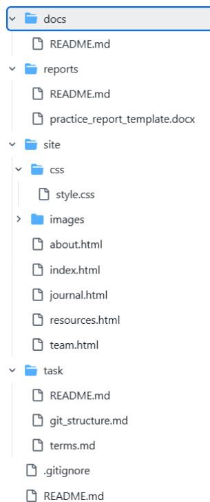
Рисунок 1 – репозиторий проекта на GitHub.
