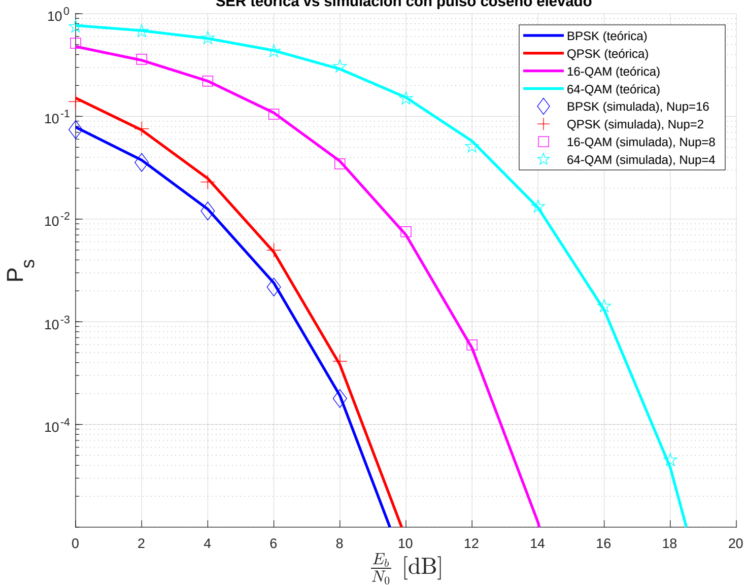
SER teórica vs simulación con pulso coseno elevado
