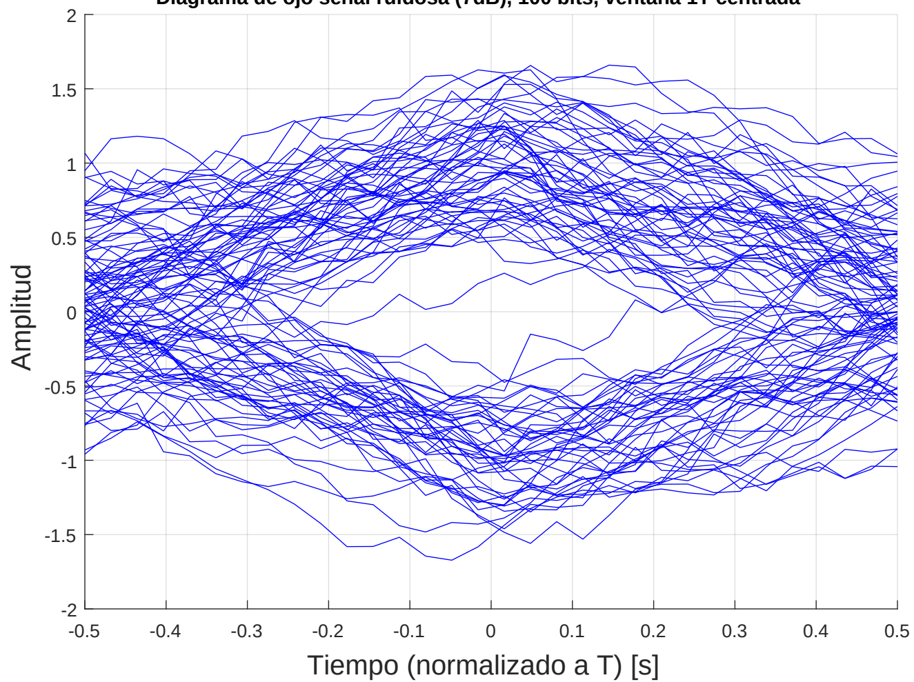
Diagrama de ojo señal ruidosa (7dB), 100 bits, ventana 1T centrada
