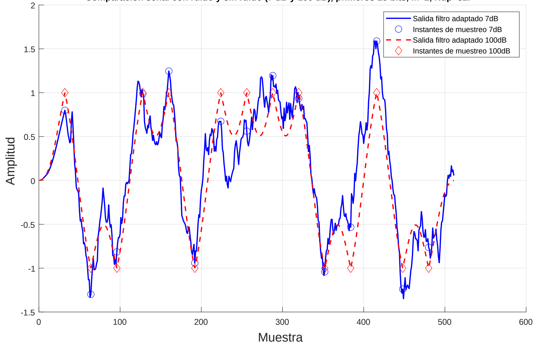
Comparación señal con ruido y sin ruido (7 dB y 100 dB), primeros 15 bits, M=2 , N_{up}=32 .
