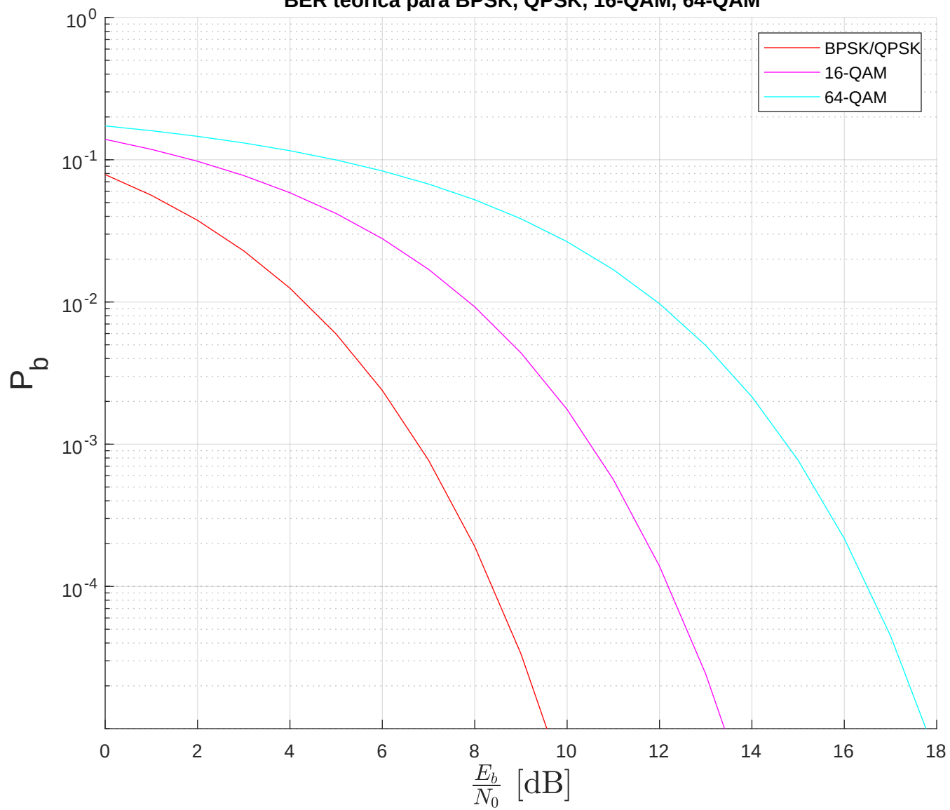
BER teórica para BPSK, QPSK, 16-QAM, 64-QAM
