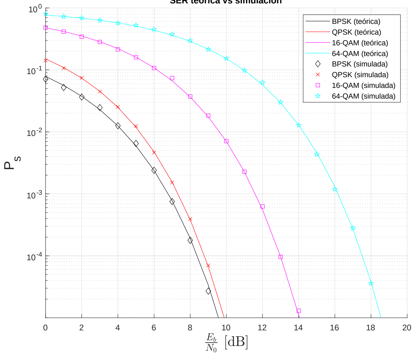
SER teórica vs simulación
