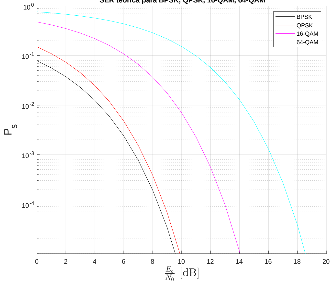
SER teórica para BPSK, QPSK, 16-QAM, 64-QAM
