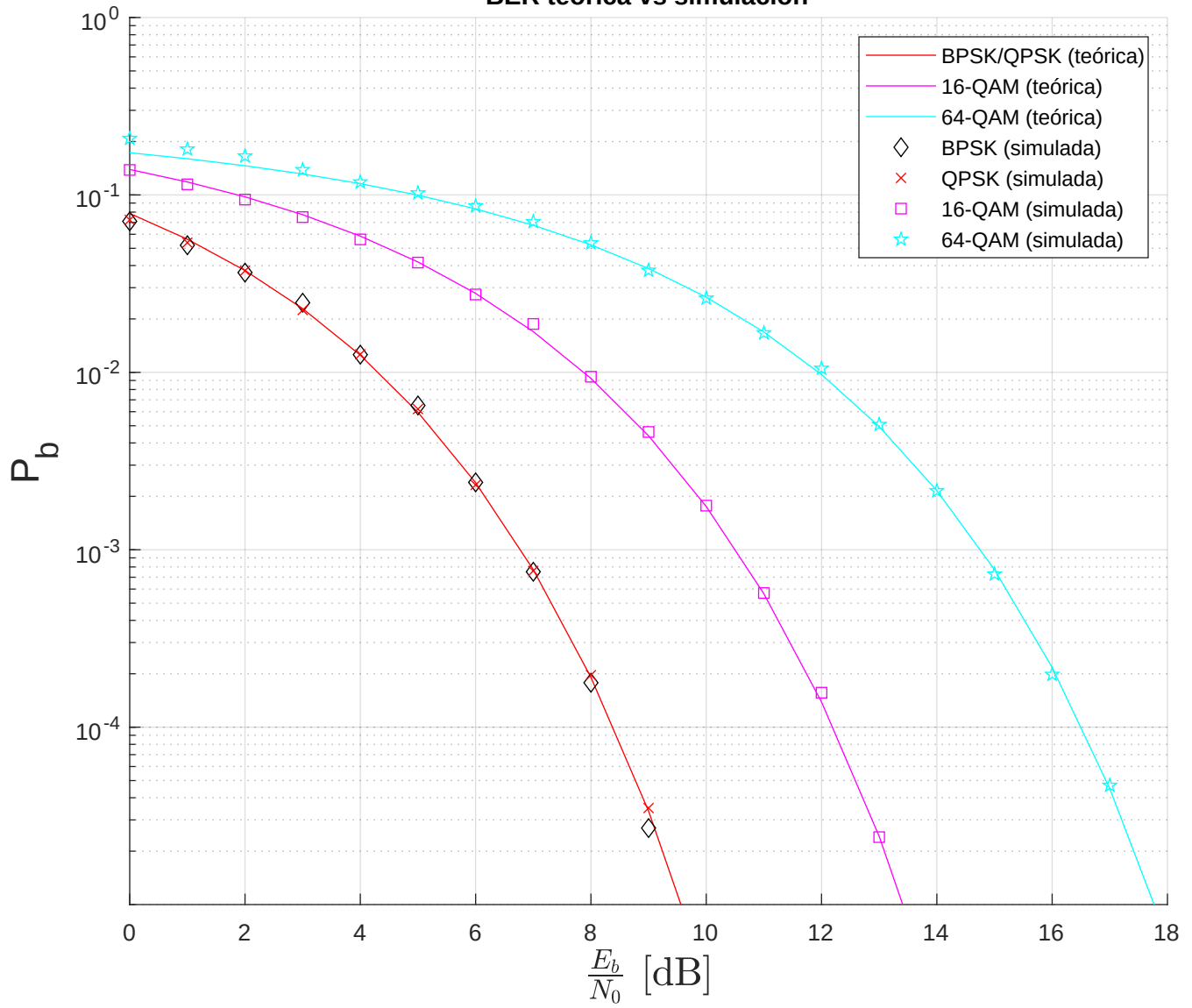
BER teórica vs simulación
