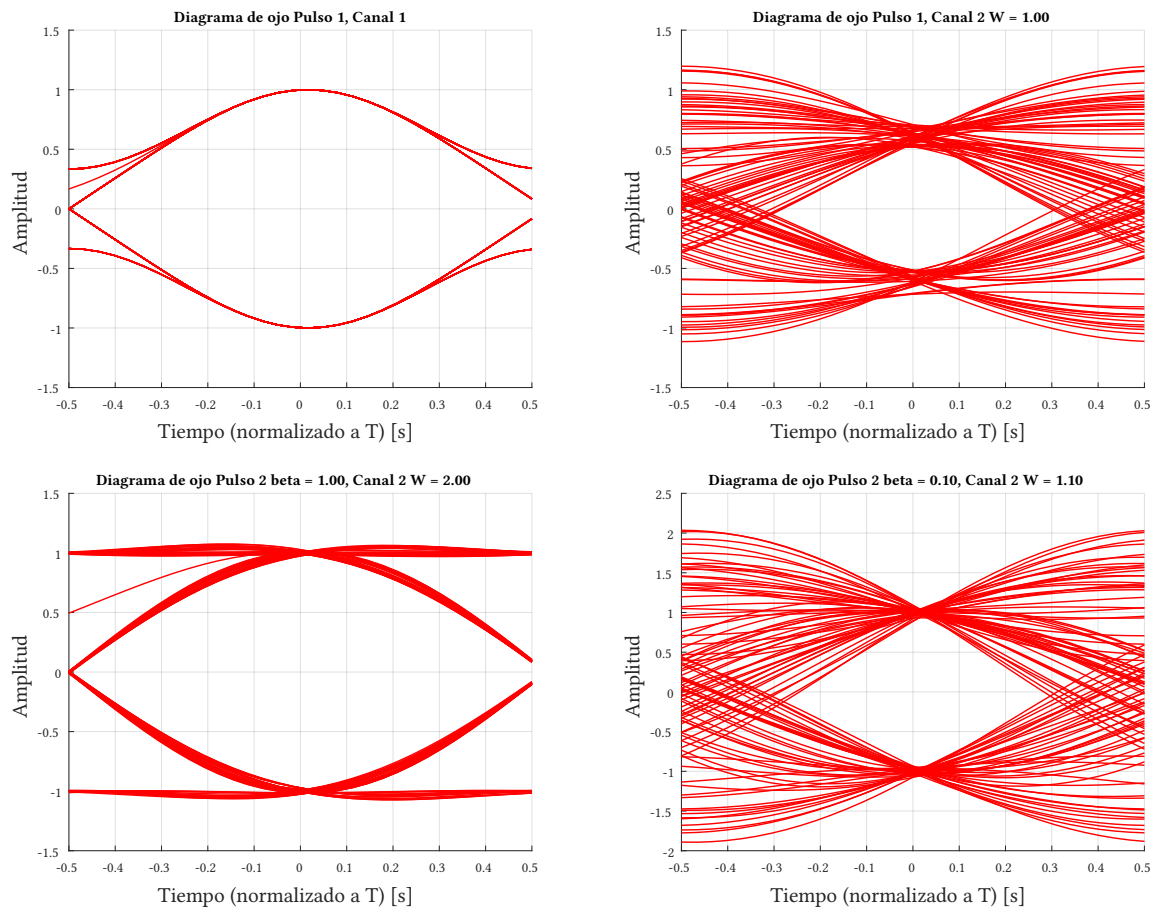
Figure 1: Comparación diagramas de ojo
