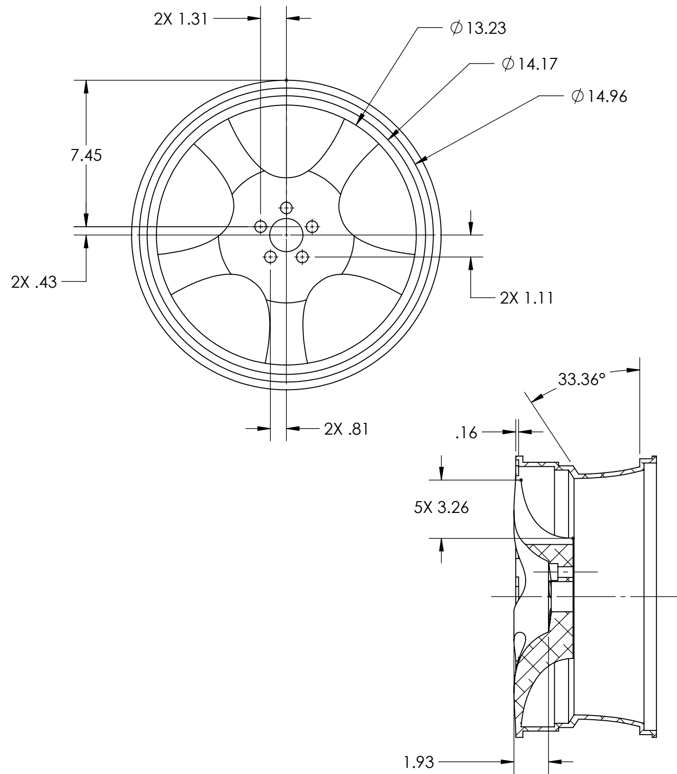
SECTION A-A SCALE 1 : 5.5
