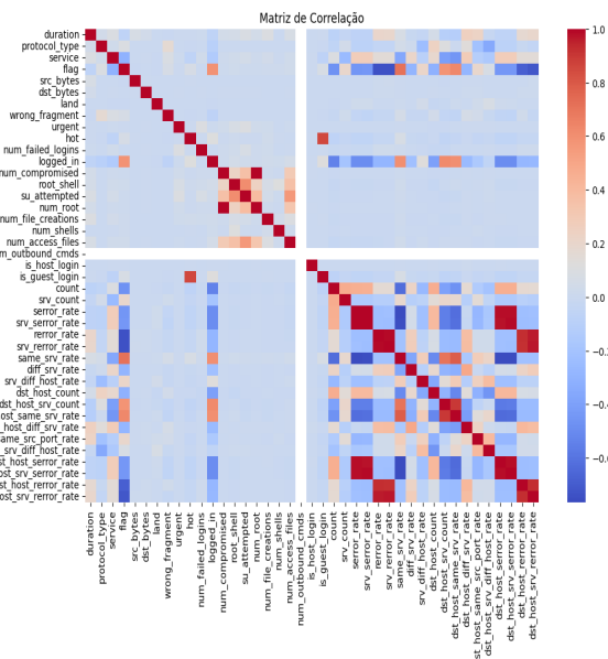
Figura 4. Matriz de correlação da base NSL_KDD
