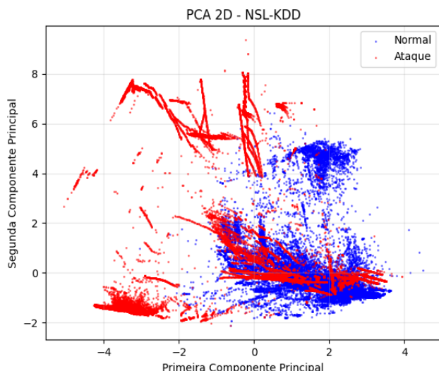
Figura 1. PCA classificando tráfego como ataque e normal
