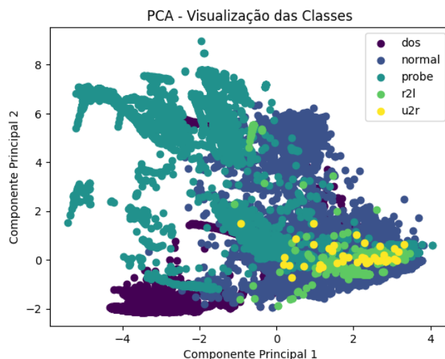
Figura 5. visualização de dois componentes do PCA separado por classes
