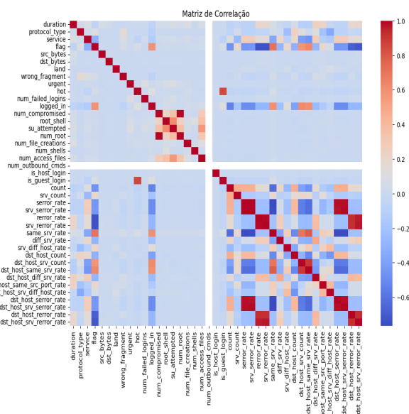
Figura 1. Matriz de correlação da base NSL_KDD
