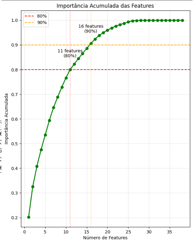
Figura 3. Representação da importância de cada feature para a acurácia
