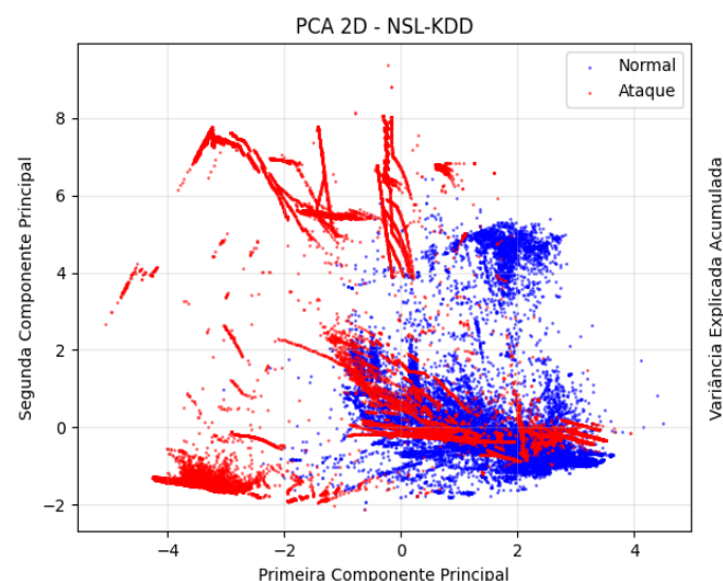
Figura 1. PCA classificando tráfego como ataque e normal
