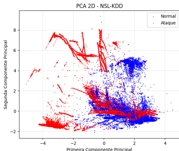
Figura 4. PCA classificando tráfego como ataque e normal
