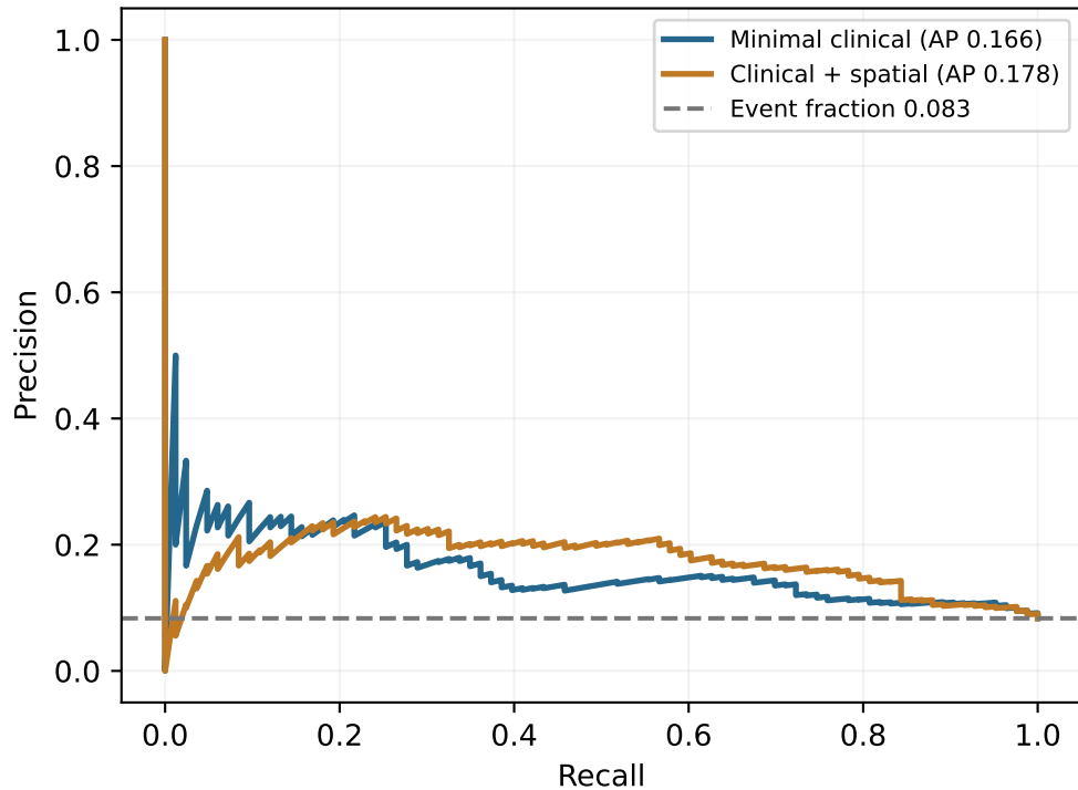
A. Precision-recall
