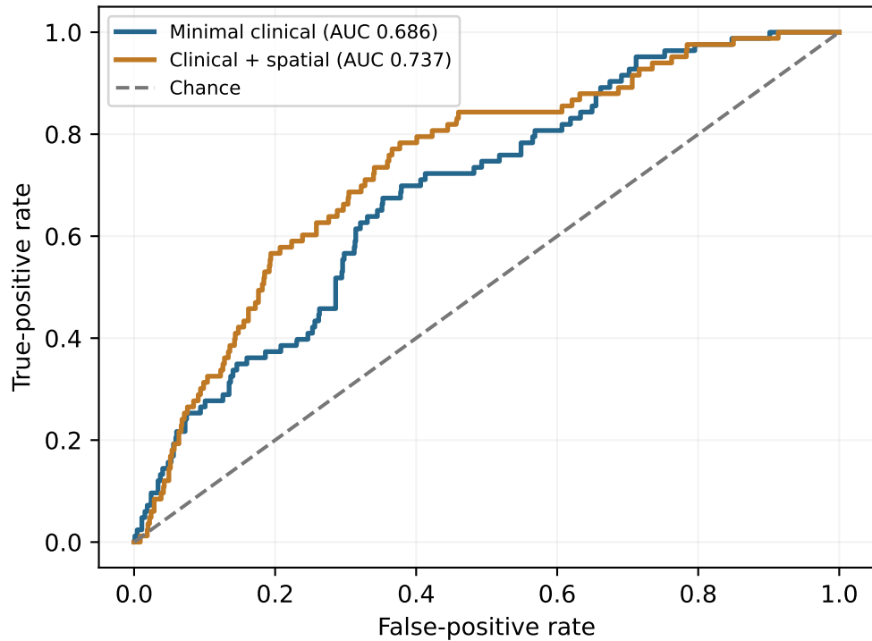
B. ROC
