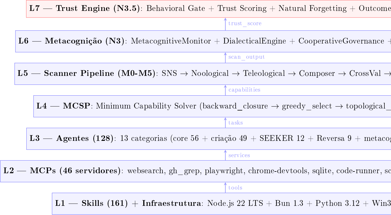
Figura 1 – Arquitetura do OpenCode Ecosystem — 7 Camadas com Fluxo de Dados
