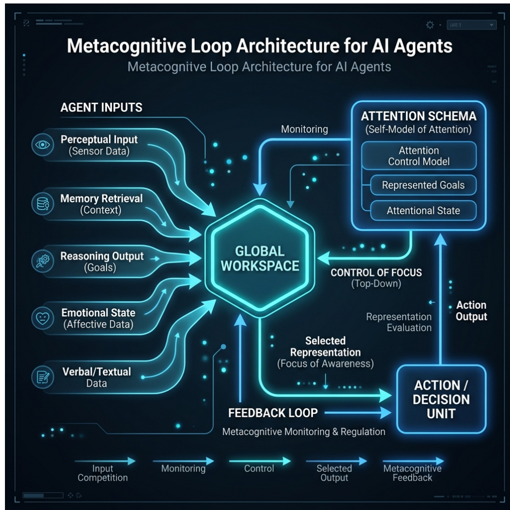
Figura 1 – Arquitetura Metacognitiva do Ecossistema baseada em GWT e AST.
