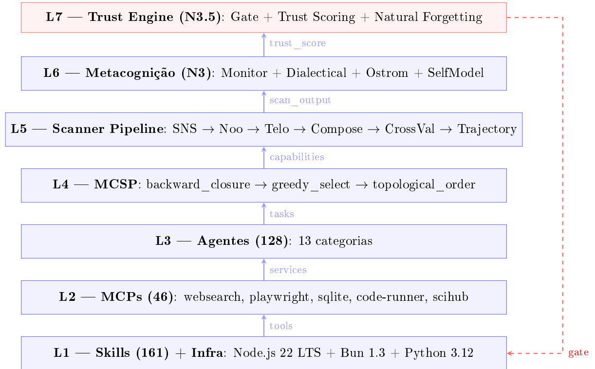
Figura 1 – Arquitetura do OpenCode Ecosystem — 7 Camadas com Fluxo de Dados
