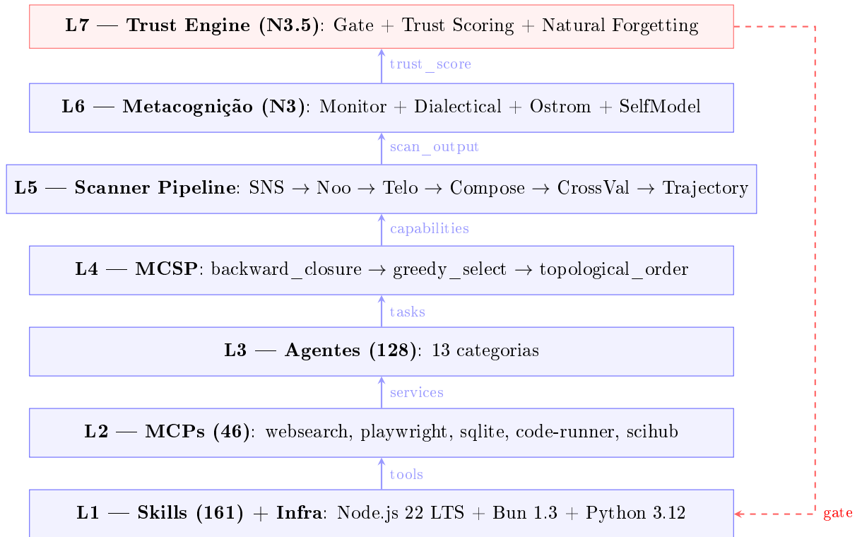
Figura 2 – Arquitetura do OpenCode Ecosystem — 7 Camadas com Fluxo de Dados
