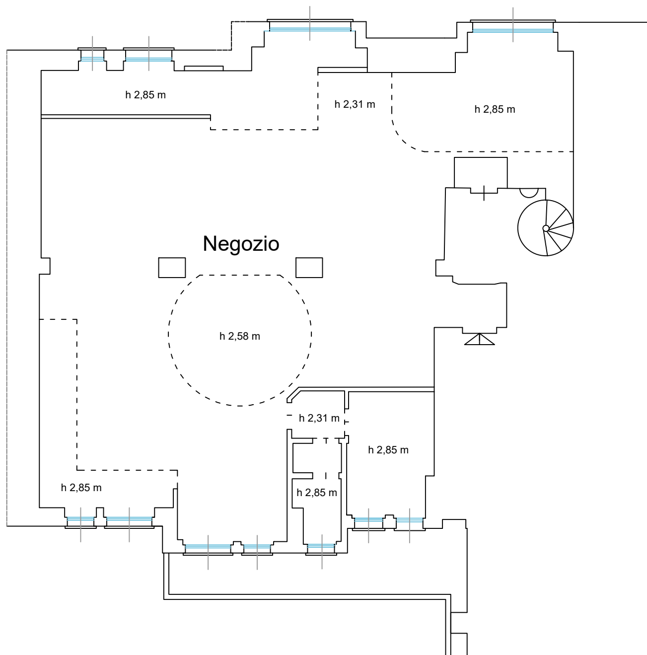
Stato di Fatto Pianta Piano Primo
