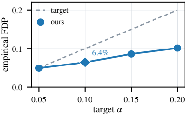
FDP
