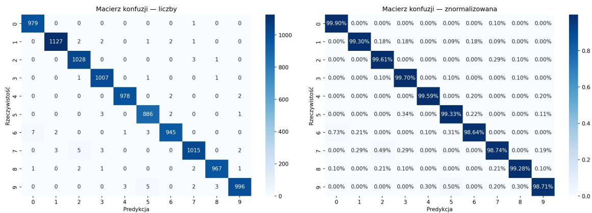
CNN MNIST — macierz konfuzji na zbiorze testowym
