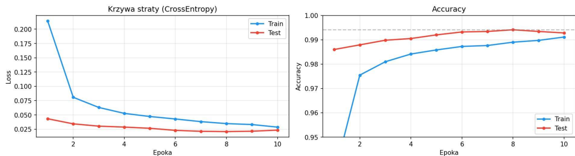
CNN MNIST — historia uczenia
