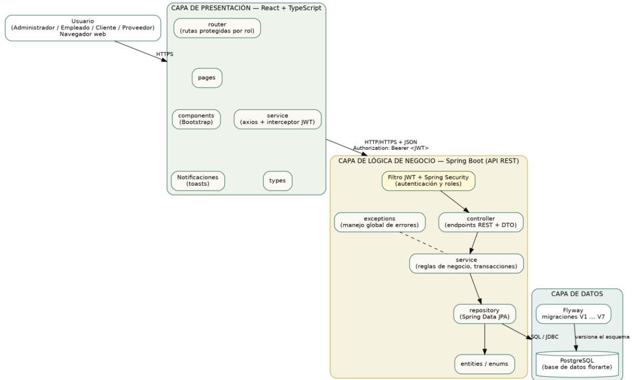
Figura 1. Arquitectura de capas del sistema Flor Arte (presentación, lógica de negocio y datos).
