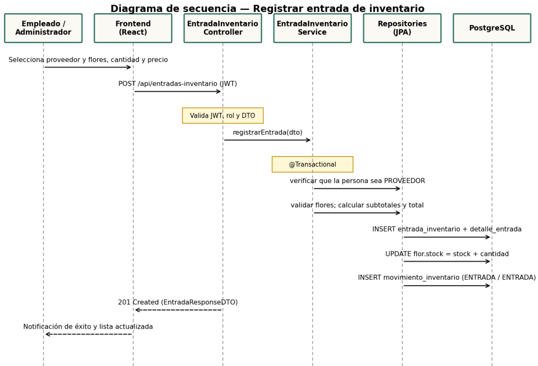
Figura 7. Secuencia de registro de entrada de inventario, con actualización automática de existencias.
