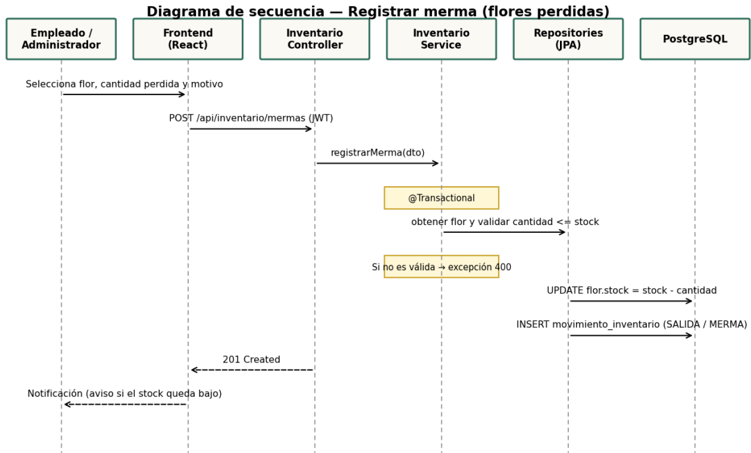
Figura 9. Secuencia de registro de pérdida (merma) de flores y actualización de inventario.
