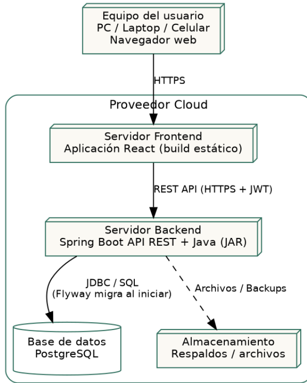
Figura 2. Diagrama de despliegue de la infraestructura Cloud de Flor Arte.
