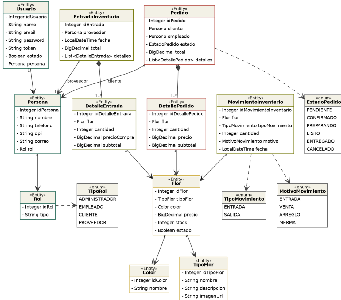
Figura 4. Diagrama de clases del dominio: entidades y enumeraciones.
