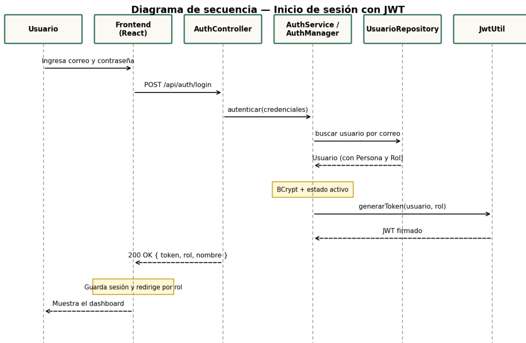
Figura 6. Secuencia de inicio de sesión: validación de credenciales y emisión del JWT.
