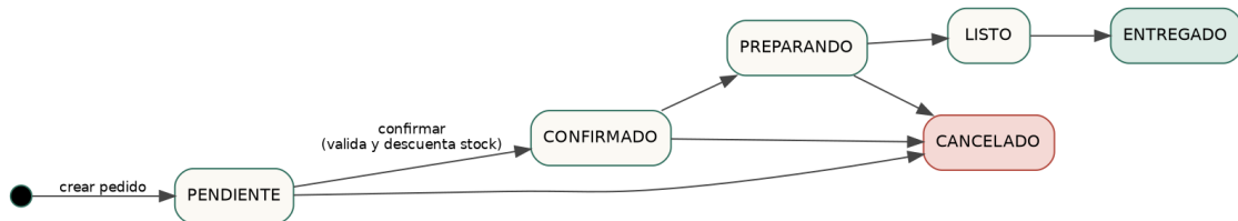
Figura 10. Ciclo de vida del estado de un pedido, de PENDIENTE a ENTREGADO o CANCELADO.
