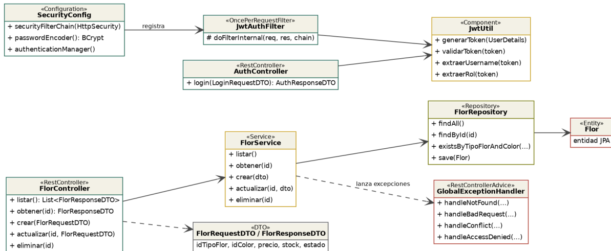
Figura 5. Relación entre Controller, Service, Repository, DTO y componentes de seguridad JWT.
