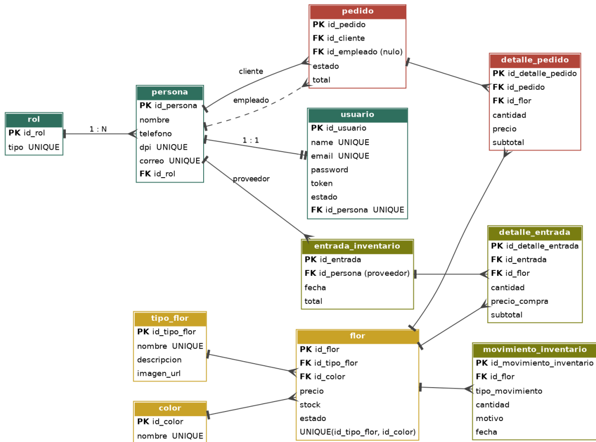
Figura 3. Modelo entidad-relación de la base de datos florarte.
