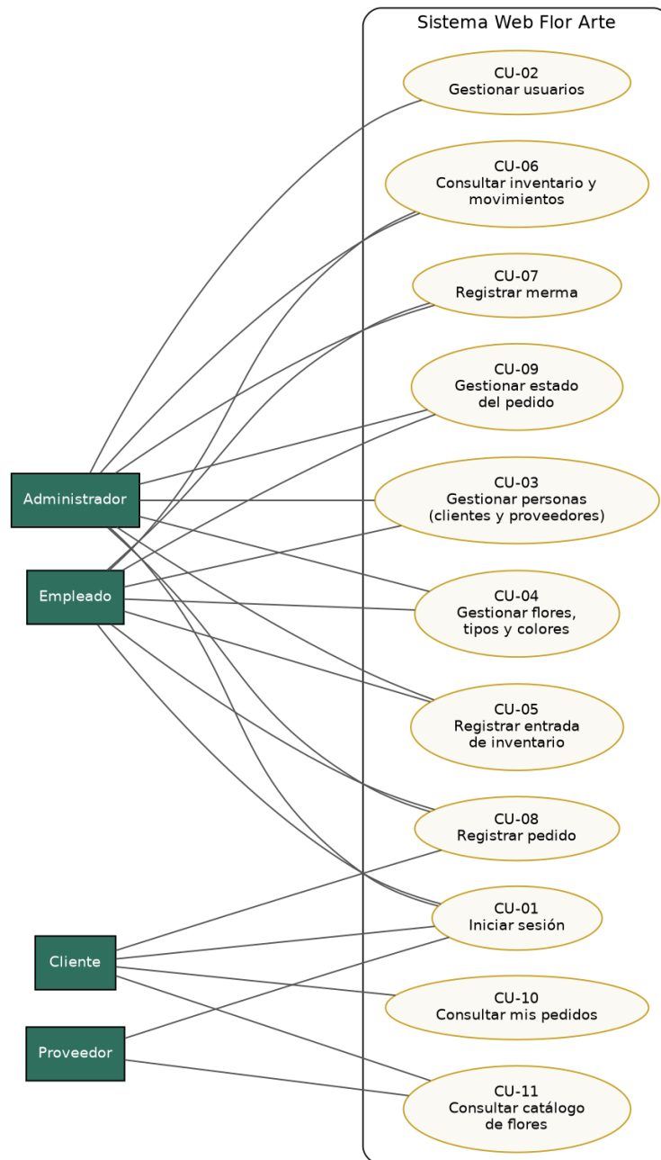
Figura 11. Diagrama de casos de uso por actor: Administrador, Empleado, Cliente y Proveedor.
