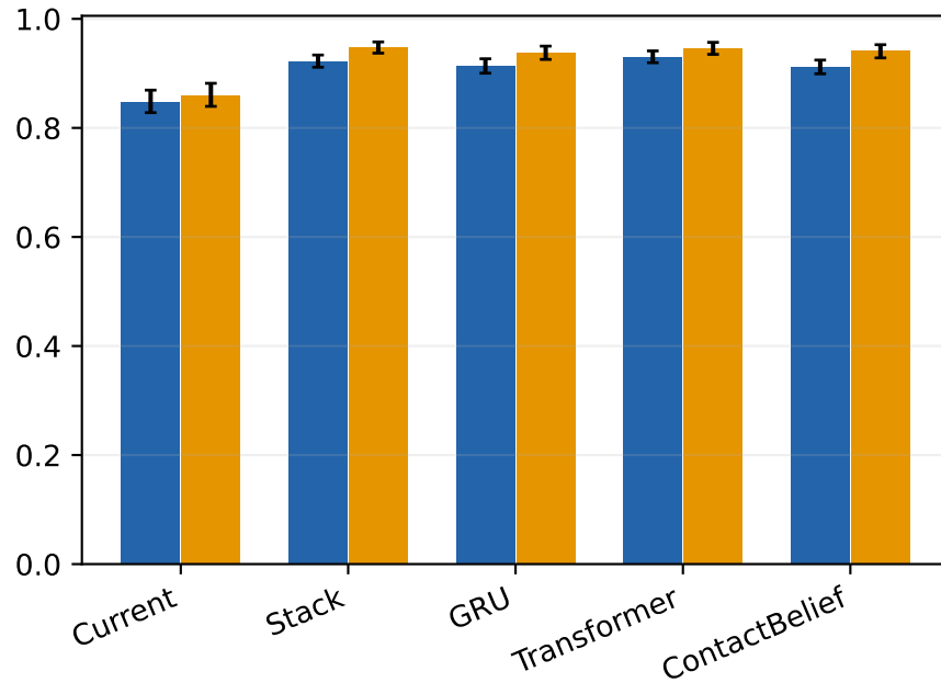
auROC
