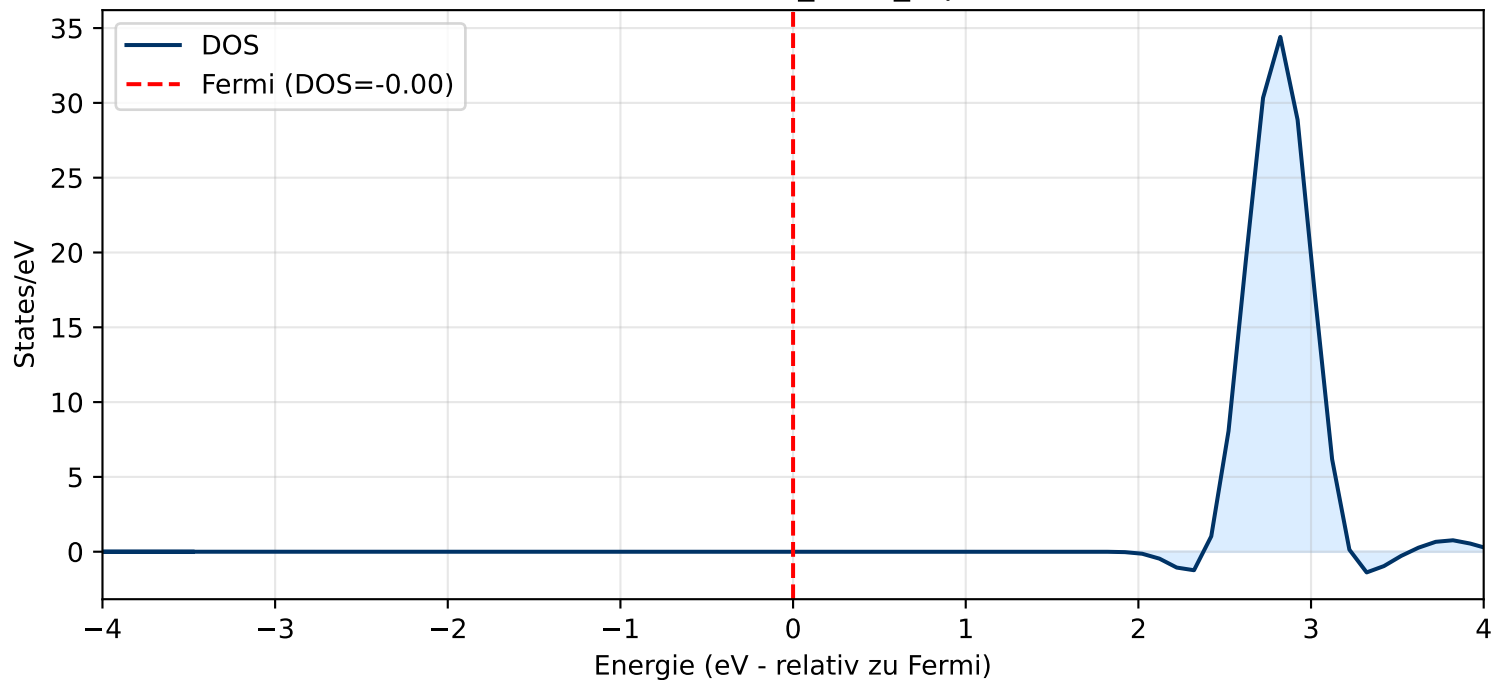
Zustandsdichte: 01_HfH3_Top1 (NEIN)
