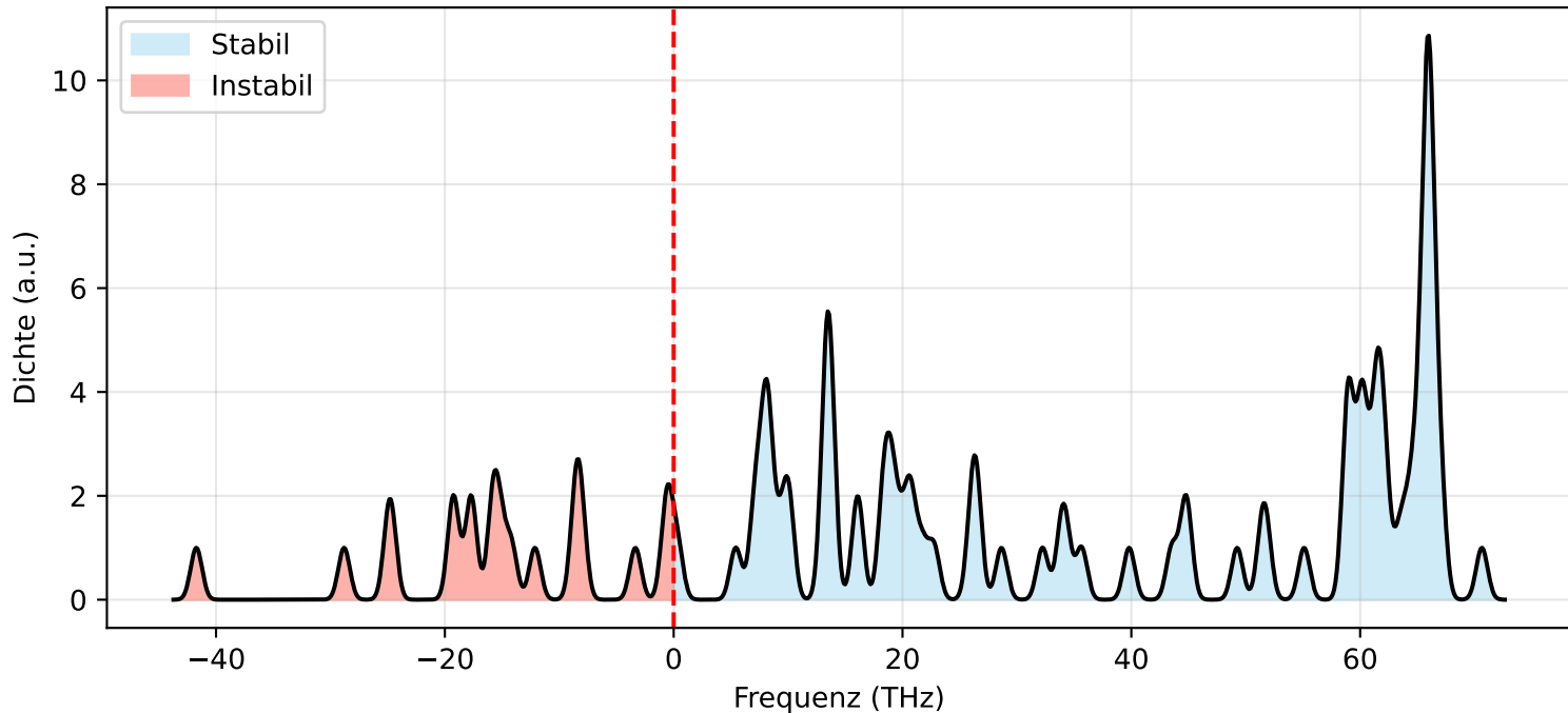
Phononen-Stabilität: 01_HfH3_Top1 (Min: -41.72 THz)
