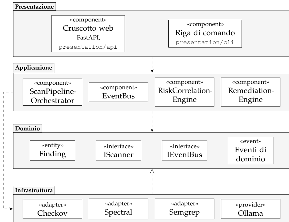
Figura 3.1: Diagramma UML dei componenti del sistema, raggruppati per livello architetturale. Le frecce tratteggiate indicano dipendenze; quella con la punta triangolare vuota indica la realizzazione delle interfacce di dominio da parte degli adapter.
