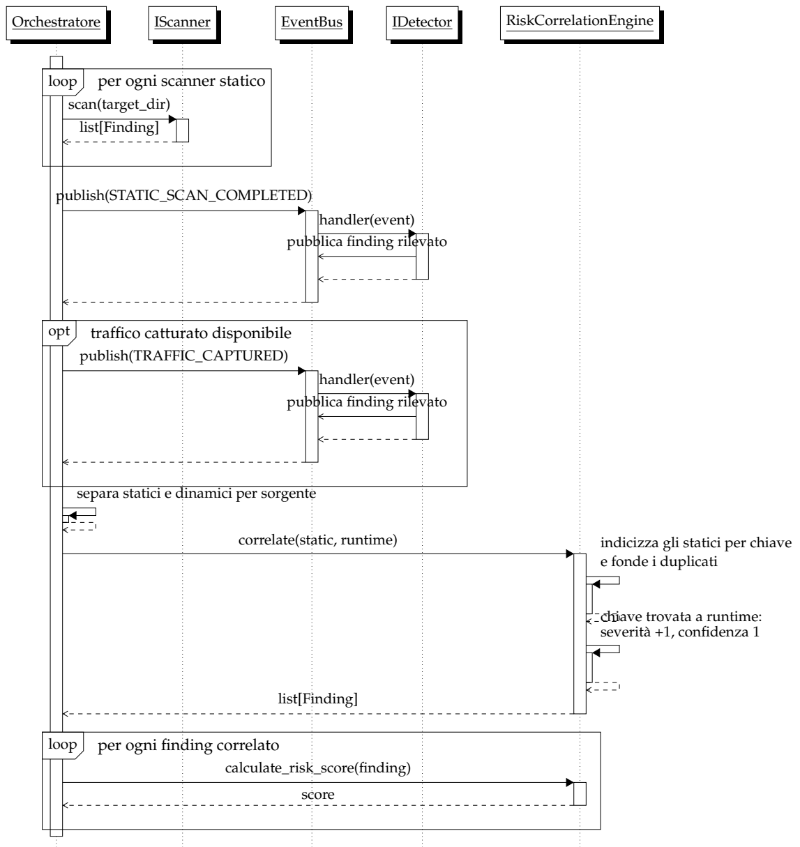
Figura 3.4: Diagramma UML di sequenza della pipeline dell’orchestratore. IScanner rappresenta gli adapter statici (Checkov, Spectral, Semgrep); IDetector i moduli che reagiscono agli eventi di completamento della scansione statica e di cattura del traffico.
