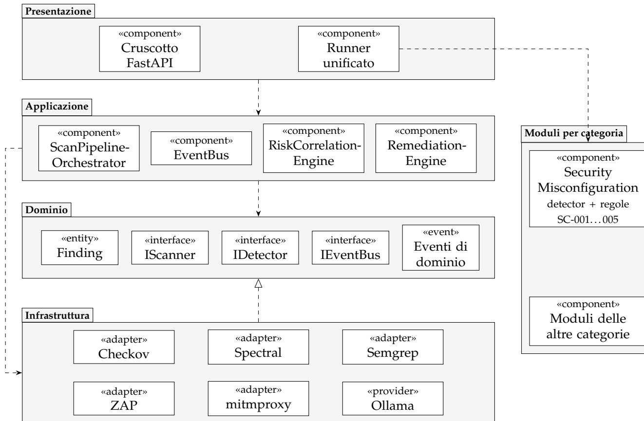
Figura 3.1: Diagramma UML dei componenti del sistema, raggruppati per livello architetturale. Le frecce tratteggiate indicano dipendenze; quella con la punta triangolare vuota indica la realizzazione delle interfacce di dominio da parte degli adapter. I moduli per categoria, fra cui quello per la Security Misconfiguration, sono invocati dal livello di presentazione e usano modelli propri.
