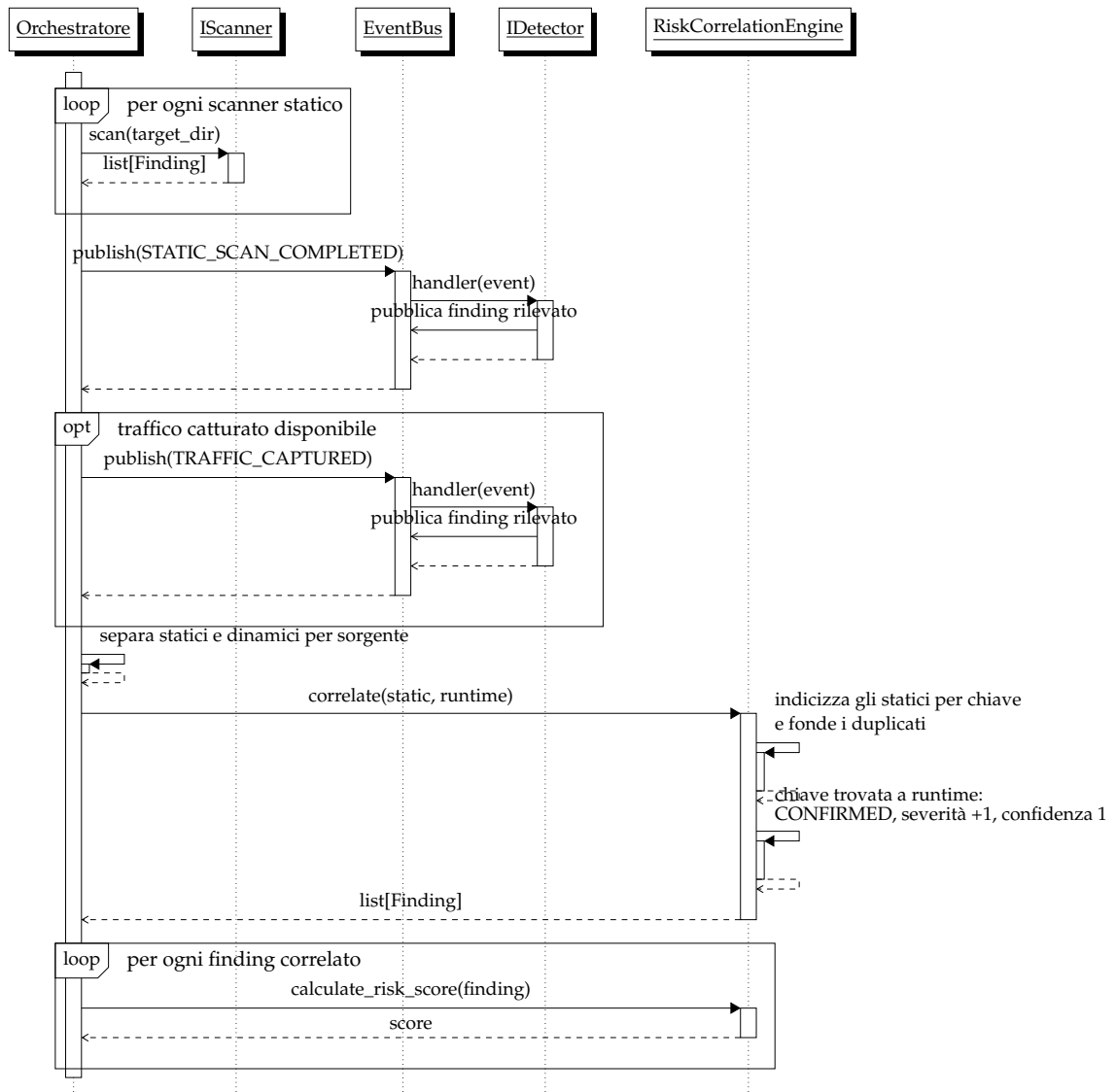
Figura 3.4: Diagramma UML di sequenza della pipeline dell’orchestratore. IScanner rappresenta gli adapter statici (Checkov, Spectral, Semgrep); IDetector i moduli che reagiscono agli eventi di completamento della scansione statica e di cattura del traffico.
