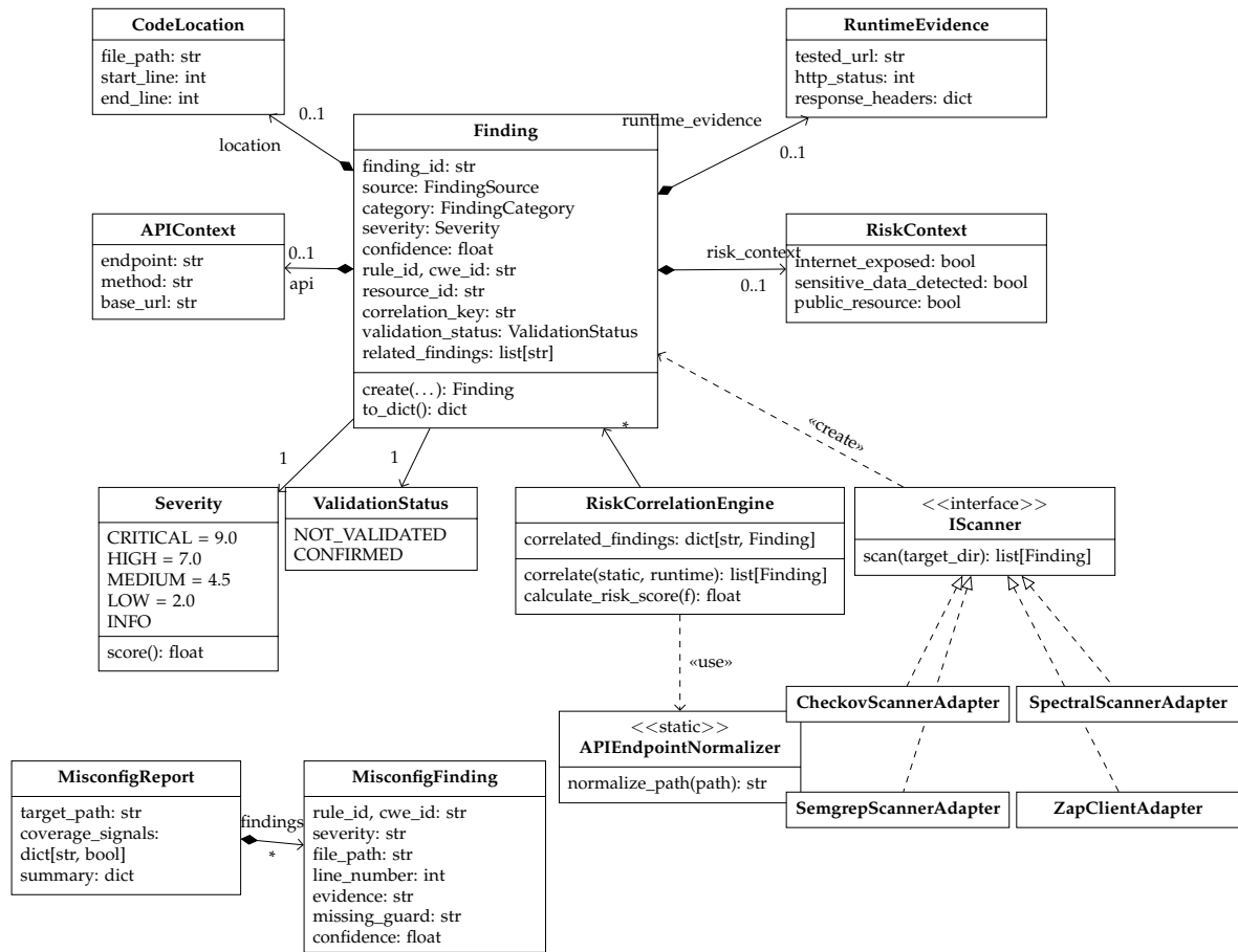
Figura 3.2: Diagramma UML delle classi del dominio e del motore di correlazione. Severity e ValidationStatus sono enumerazioni; APIEndpointNormalizer espone solo metodi di classe. In basso a sinistra i modelli del modulo per la Security Misconfiguration, che non derivano da Finding .
