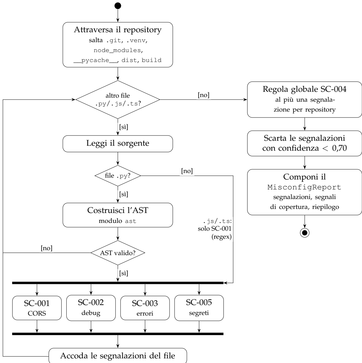
Figura 3.3: Diagramma UML di attività della funzione analyze del modulo di analisi del codice applicativo. Le quattro regole locali sono invocate su ogni file; la regola globale SC-004 e il filtro di confidenza operano una sola volta, a valle del ciclo.
