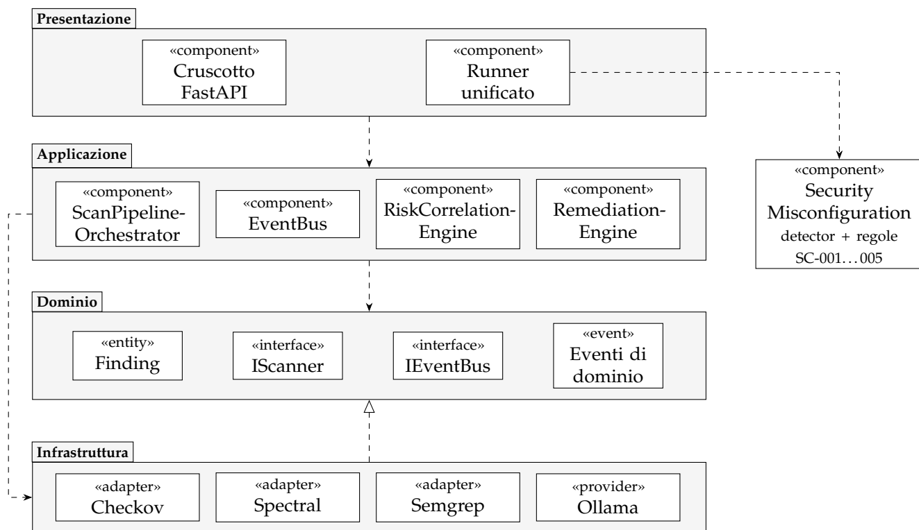
Figura 3.1: Diagramma UML dei componenti del sistema, raggruppati per livello architetturale. Le frecce tratteggiate indicano dipendenze; quella con la punta triangolare vuota indica la realizzazione delle interfacce di dominio da parte degli adapter. Il modulo per la Security Misconfiguration è invocato dal livello di presentazione e usa modelli propri.
