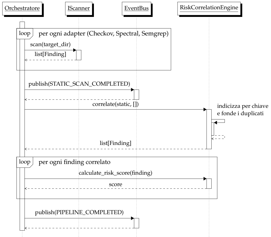
Figura 3.4: Diagramma UML di sequenza della pipeline statica dell’orchestratore. IScanner rappresenta gli adapter Checkov, Spectral e Semgrep; il secondo argomento di correlate , riservato alle segnalazioni a runtime di altri moduli, è vuoto.
