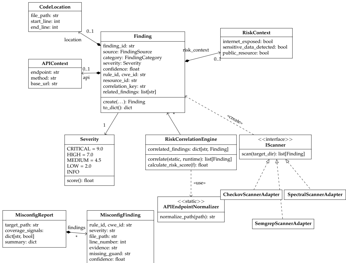
Figura 3.2: Diagramma UML delle classi del dominio e del motore di correlazione. Severity è un'enumerazione; APIEndpointNormalizer espone solo metodi di classe. In basso a sinistra i modelli del modulo per la Security Misconfiguration, che non derivano da Finding .
