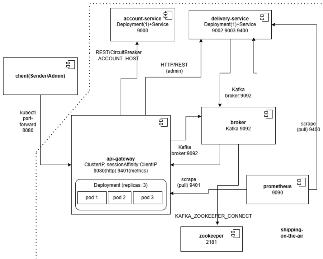
C&C di Deployment Kubernetes
