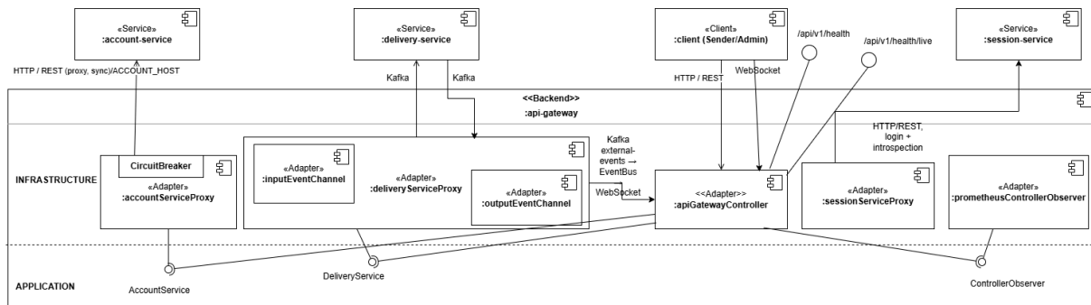
C&C dell'api-gateway
