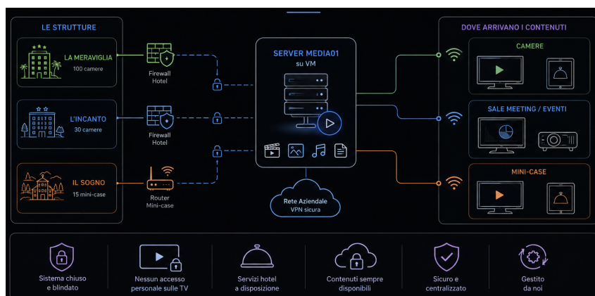
Figura 4 - Modello di distribuzione dei contenuti verso camere, sale meeting e mini-case.
