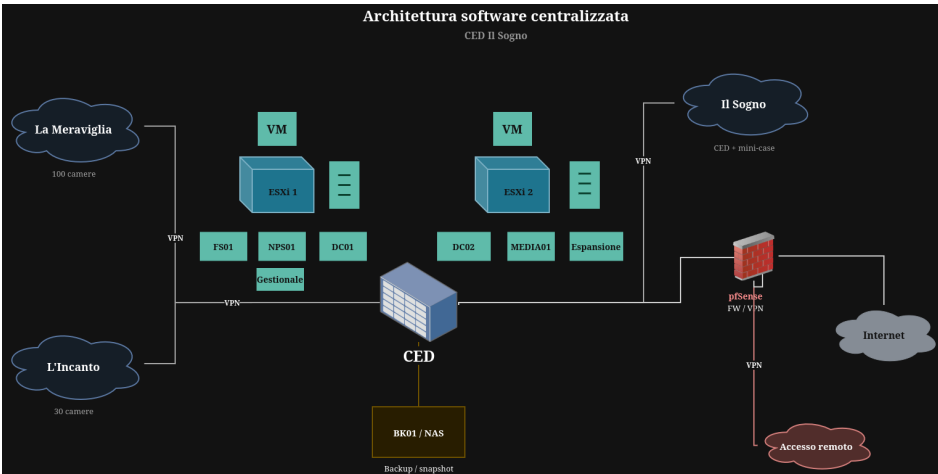
Figura 3 - Integrazione dei servizi Windows nell'architettura centralizzata del CED.
