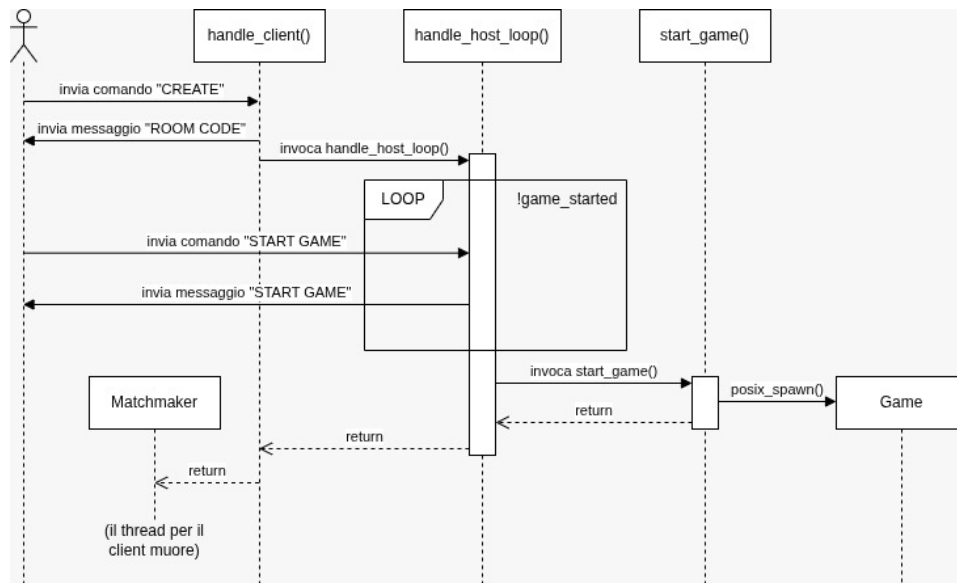
Figura 2: Processo di creazione partita e ciclo handle_host_loop
