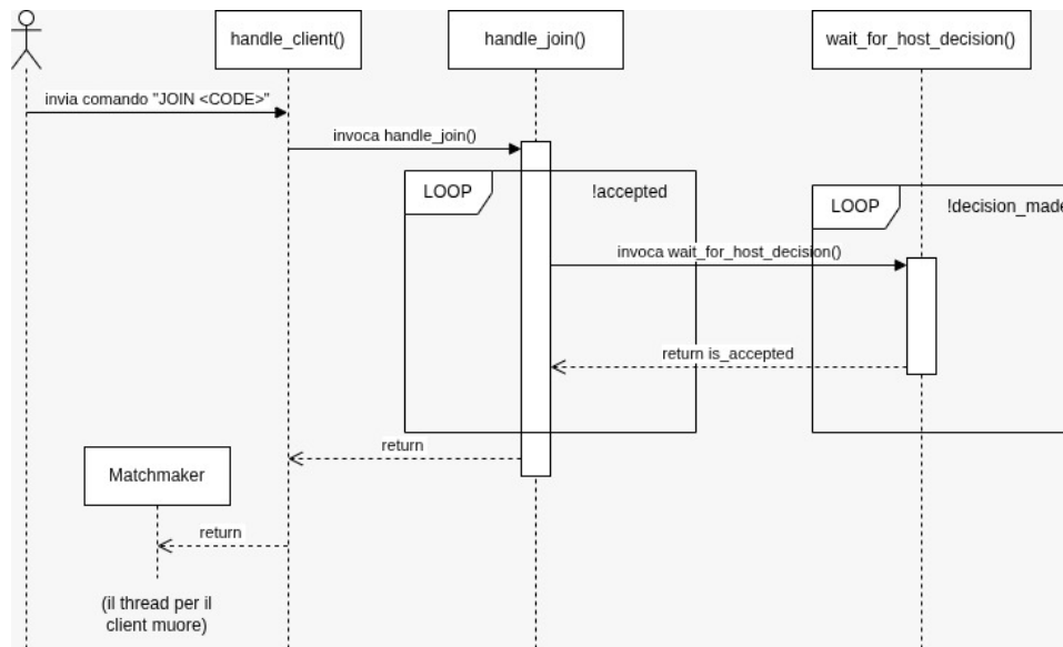
Figura 3: Processo di unione a una stanza esistente
