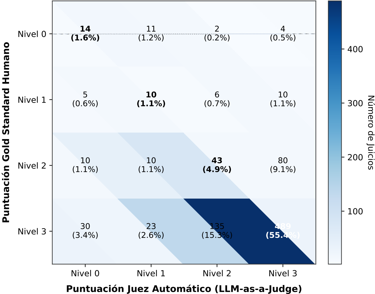
Matriz de Confusión Global: Gold Standard vs LLM-as-a-Judge ( N_K = 882 )
