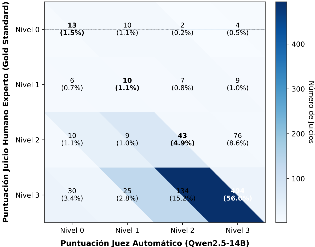
Matriz de Confusión Global: Humano vs Juez ( N_K = 882 )
