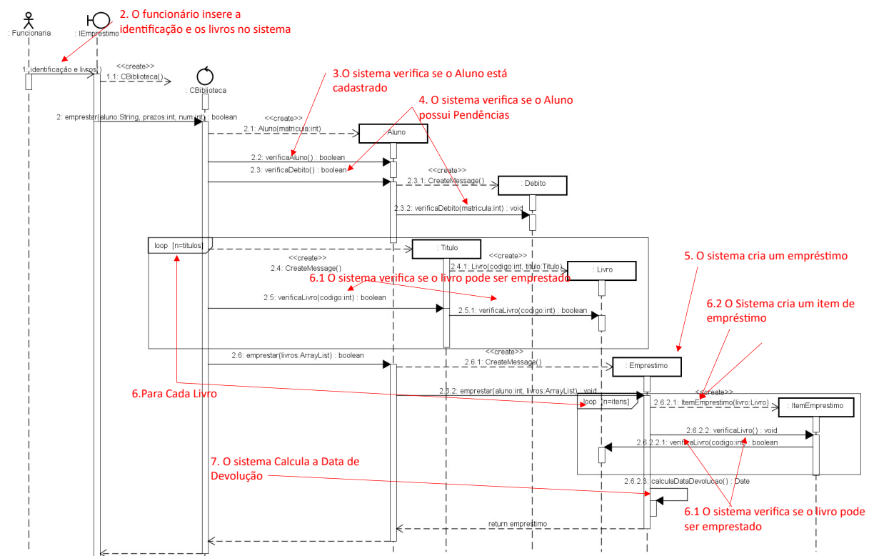
Figura 11.11: Diagrama Sequência do Empréstimo de Livro
