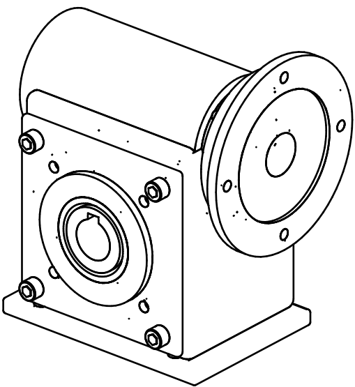
MONTADO · ESC. 1:3
