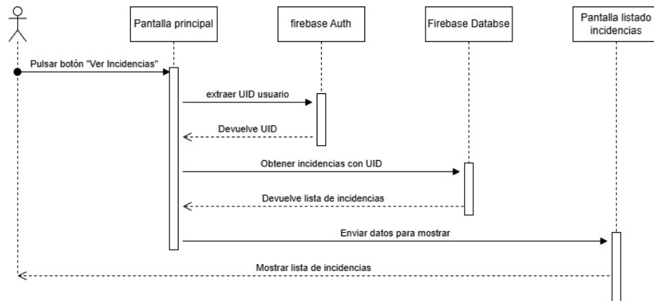
Figura C.14: Diagrama de secuencia UML ver lista de incidencia
