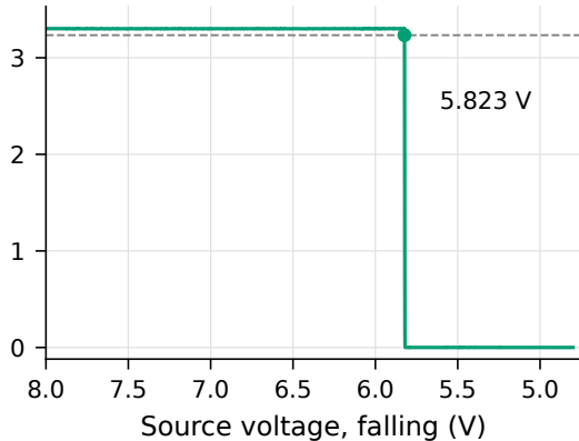
(b) 3.3 V mode
